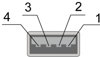
Рис. 3.7 Универсальный разъем
