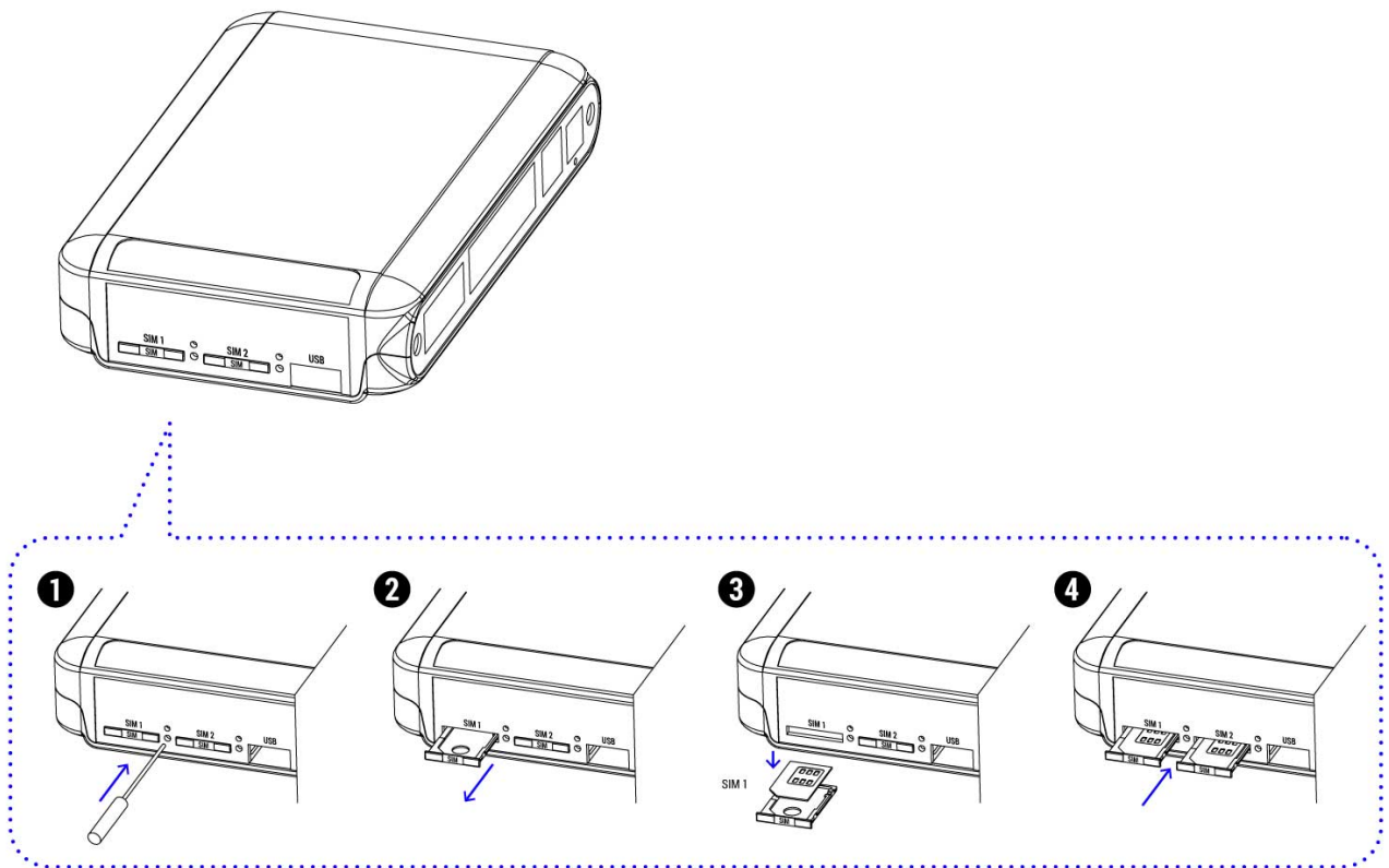
Рис. 4.1 Установка SIM-карт
